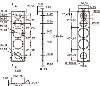
面板
