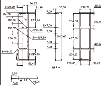
面网板
